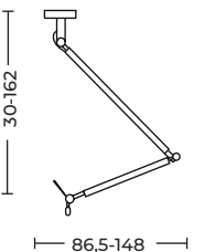
ZYTA M PENDANT LAMPBODY AZ2304
