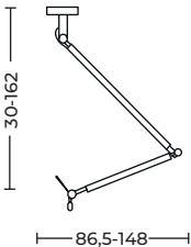
ZYTA M PENDANT LAMPBODY AZ4192
